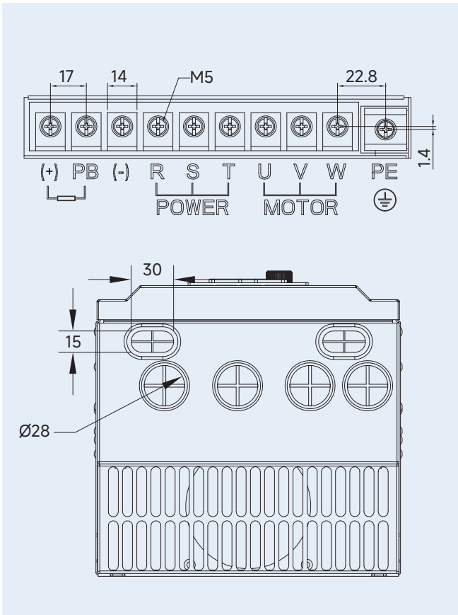
a) Applies to RNB2015 ~ RNB2022
